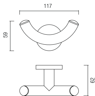
BA 715 - Double Robe Hook
